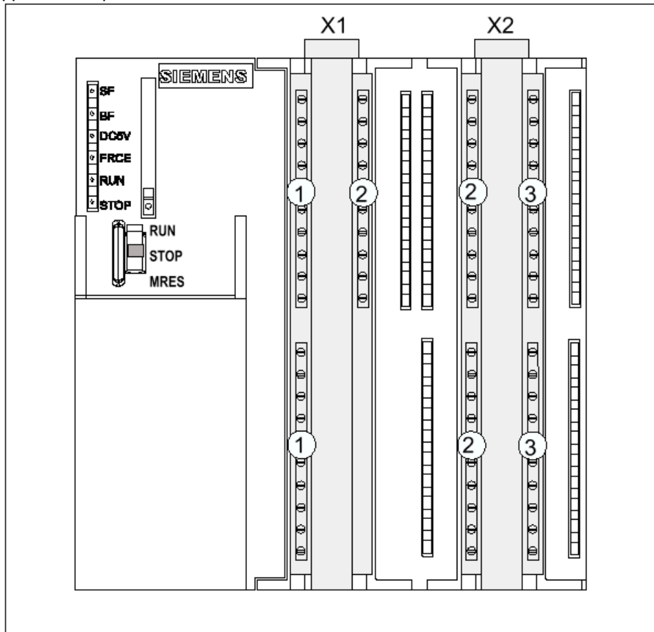
Рис. 3-2. Встроенные входы и выходы CPU 31xС (напр., CPU 314C-2 PtP)
