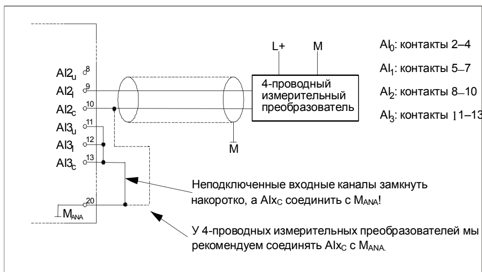
Рис. 7-8. Подключение 4-проводного измерительного преобразователя к аналоговому токовому и потенциальному входу CPU 313C/314C-2
